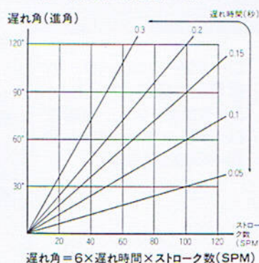
エアリーリースにおけるシリンダの遅れ時間と遅れ角(進角)の関係
