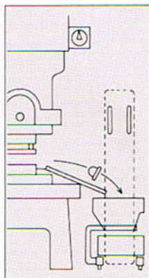
①センサ入力・シャッター連動 Sensor-shutter interlocking operation.
