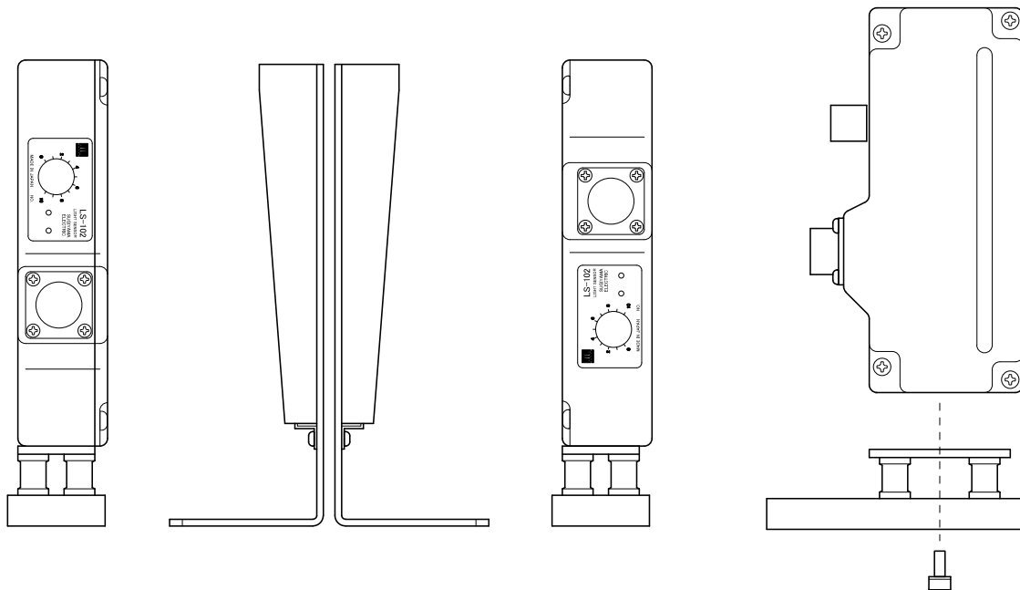
LS-102 2個取り検出使用例
