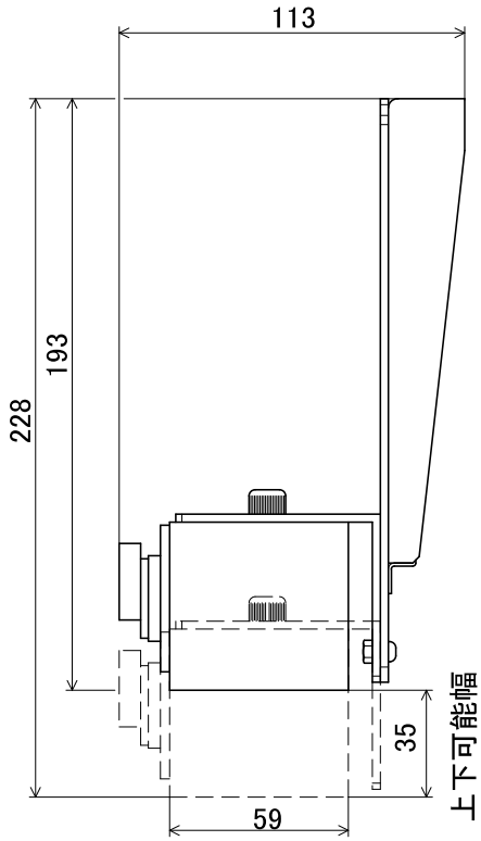
LS-102M用反射板
